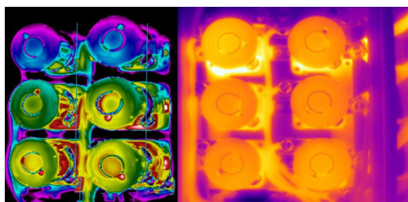
Warmtebeeld van een verdeler met zekeringshouders
